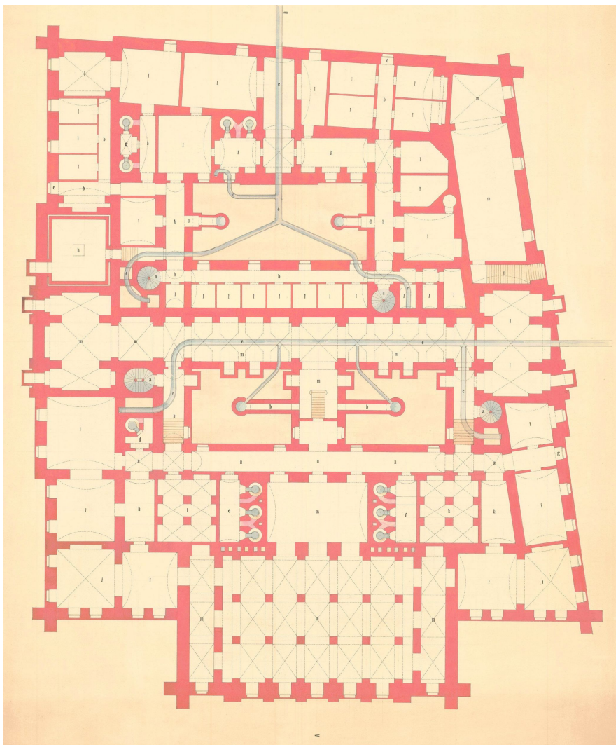
Az engedélyezési terv – pince és alagút
