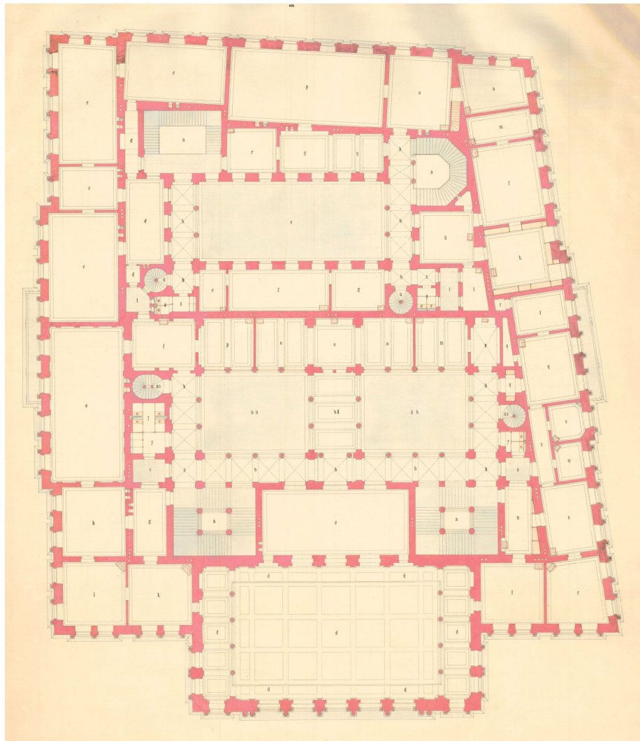
Az engedélyezési terv – 1. emelet
