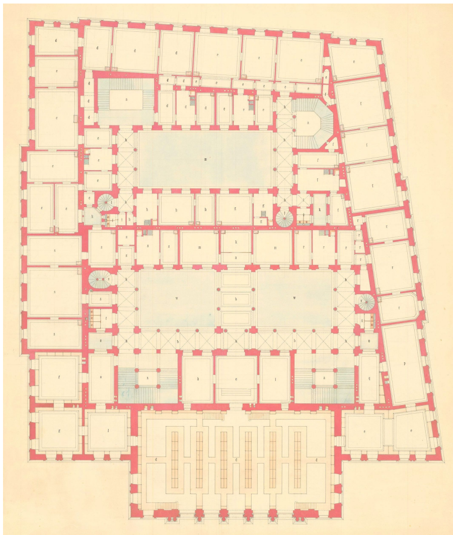
Az engedélyezési terv – 2. emelet
